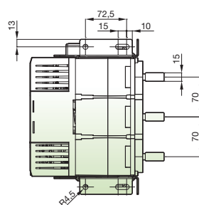
Тип V (вертикальные выводы)
