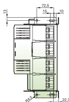
Тип Р (подключение спереди)
