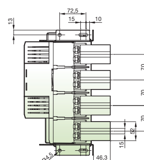
Тип Т (переднее присоединение с переходом вертикальный тип)
