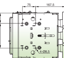
Тип Z (переднее присоединение с переходом расширенный тип)
