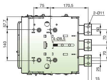
Тип Н (горизонтальные выводы)
