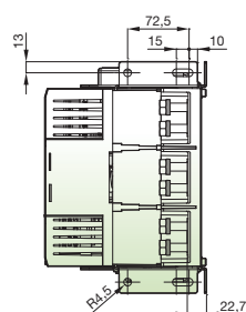
Тип P (подключение спереди)
